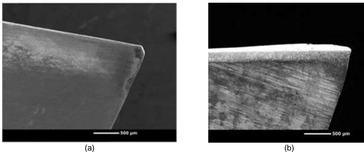
Fig. 9: Micrografías de SEM de los buriles luego del proceso de cilindrado: a) Buril sin recubrir; b) Buril recubierto con HfN.
