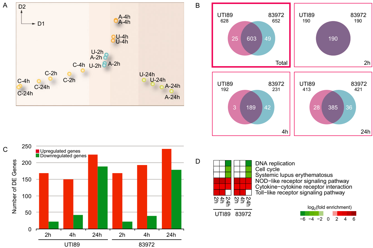
Fig. 1. BMM transcriptome analysis.
