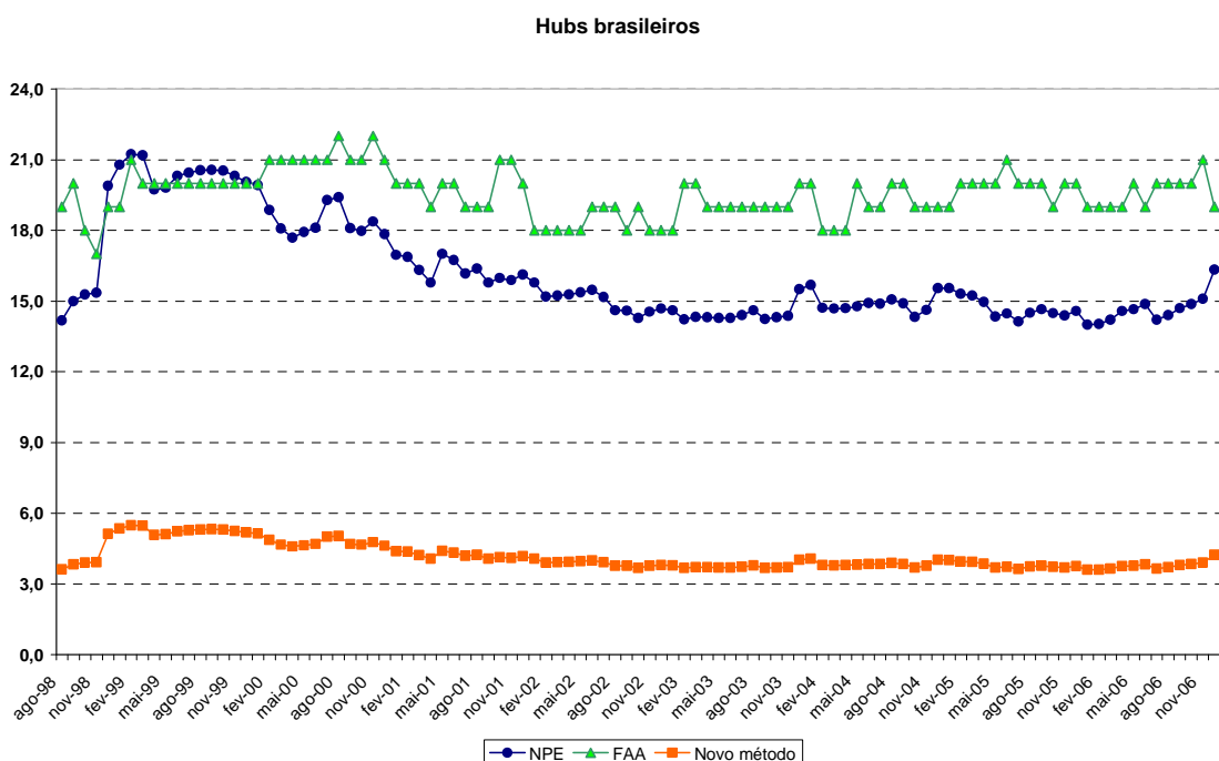
Figura 4: Número de hubs em cada período do ano de acordo com os três métodos
